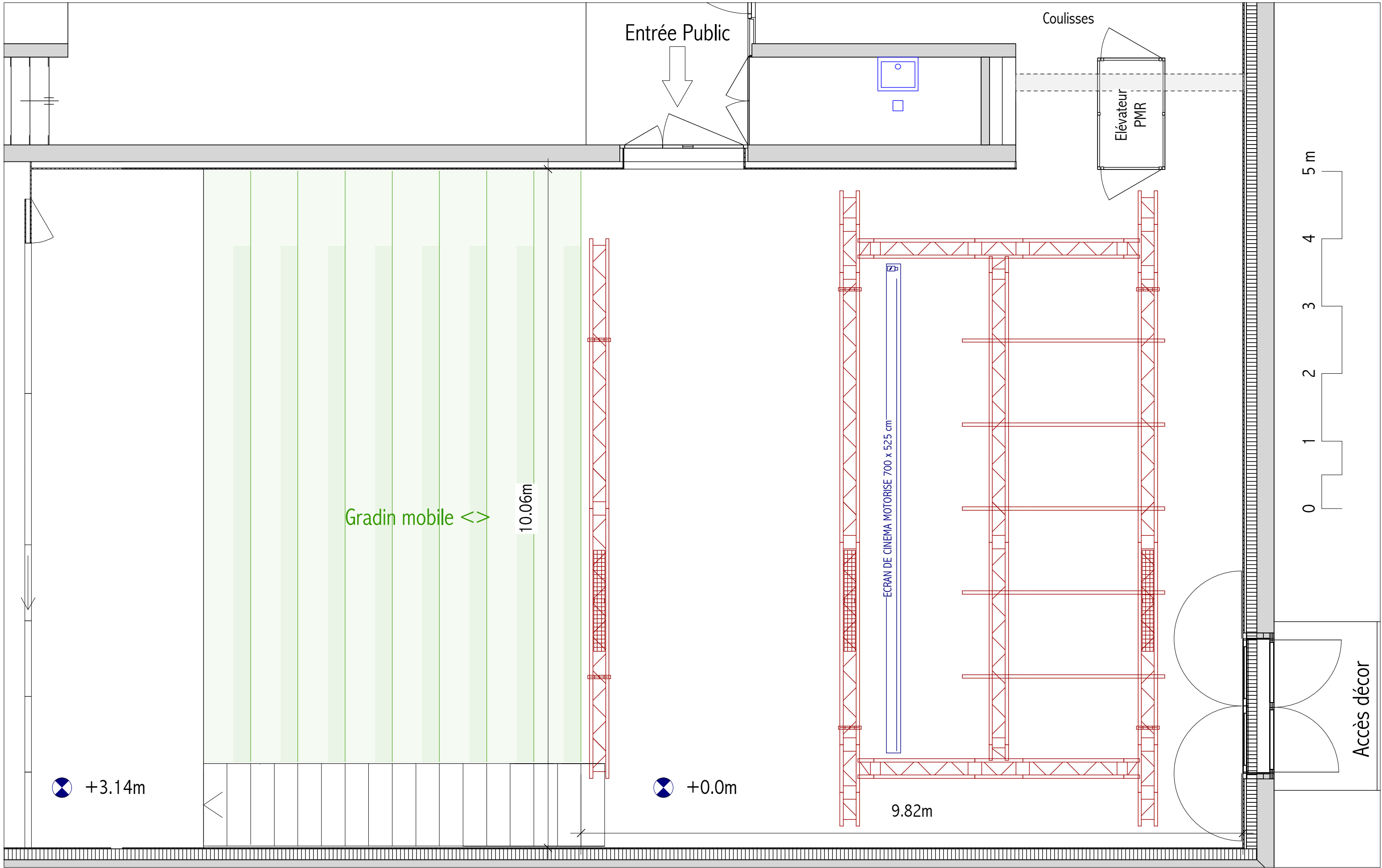
Maison de Quartier de Chailly Plan Salle de spectacle Ech.: 1/50 A3
